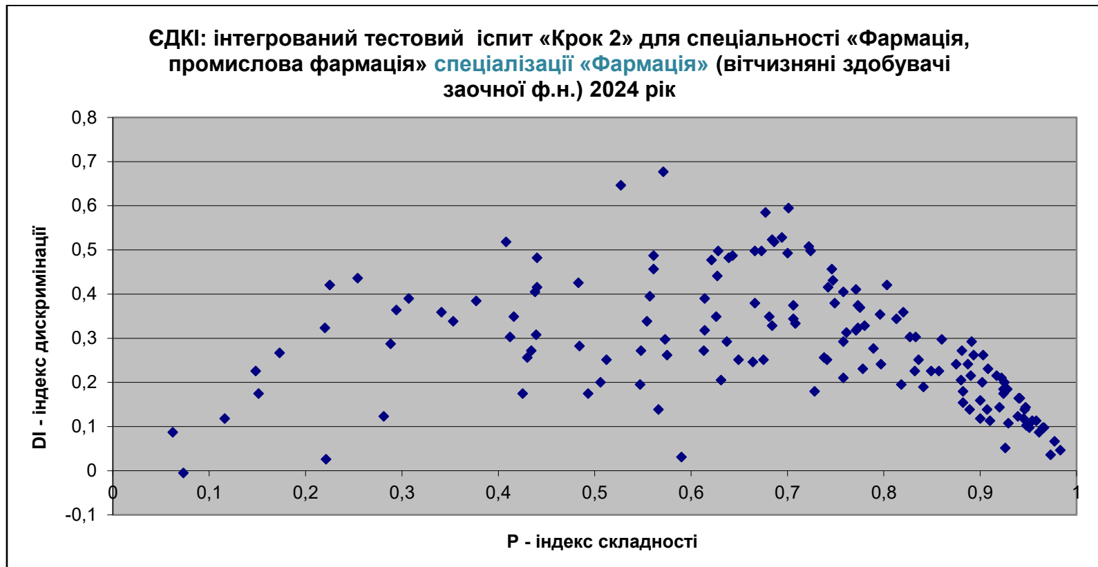
Рисунок 5. Діаграма психометрії тестових завдань ЄДКІ «Крок 2» для спеціальності «Фармація, промислова фармація» спеціалізації «Фармація»
