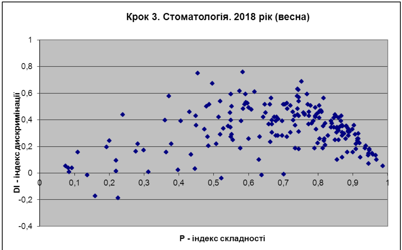
Рисунок 1. Діаграма психометрії тестових завдань ліцензійного іспиту «Крок 3. Стоматологія». 27.03.2018 (горизонтальна вісь – індекс складності, вертикальна вісь – індекс дискримінації)
