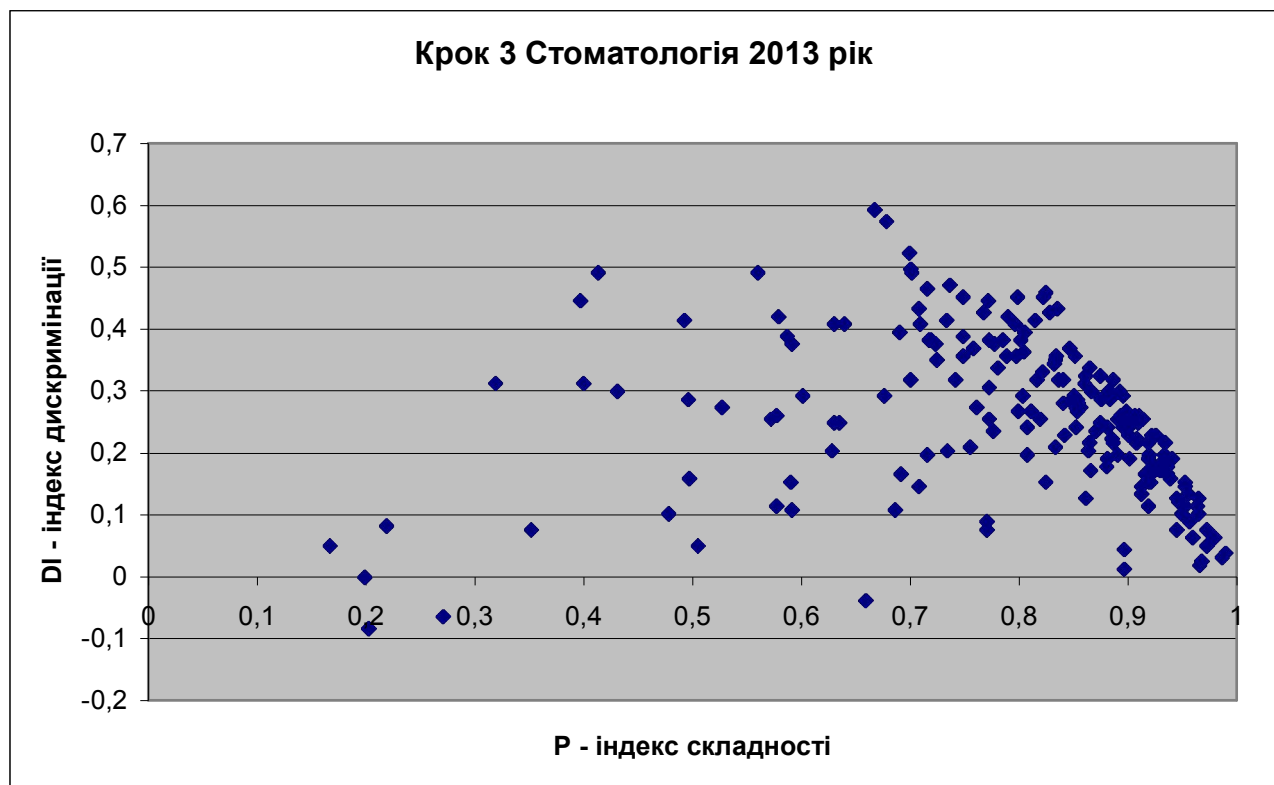
Рисунок 1. Діаграма психометрії тестових завдань Крок 3. Стоматологія. 26.03.2013 (горизонтальна вісь – індекс складності, вертикальна вісь – індекс дискримінації)
